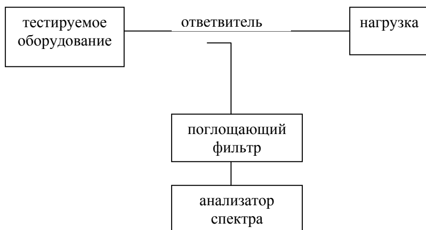
Рис. 7 Схема рабочего места для измерения паразитных излучений на антенном фланце на частотах выше критической частоты волновода.
